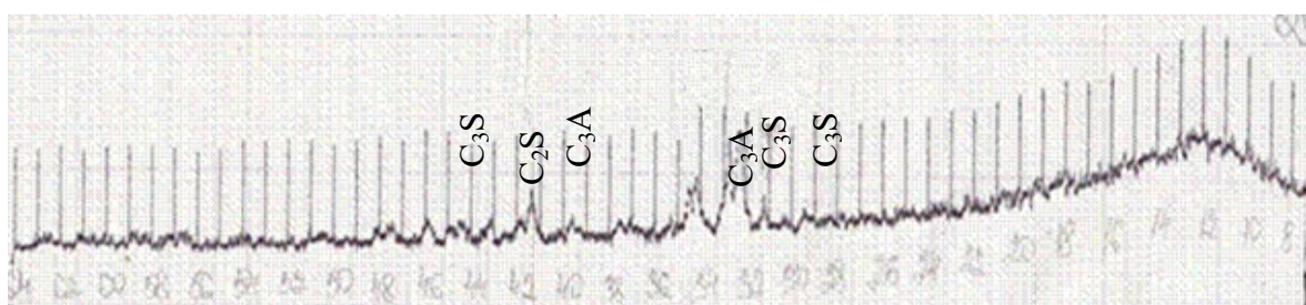
Рис. 4. Рентгенограмма синтезированного цементного клинкера
