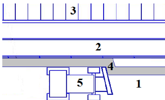
Рис. 3. Пододвигание корма: 1 – кормовой стол, 2 – навозный канал, 3 – секция для содержания дойных коров, 4 – корм, 5 – трактор с ковшем
