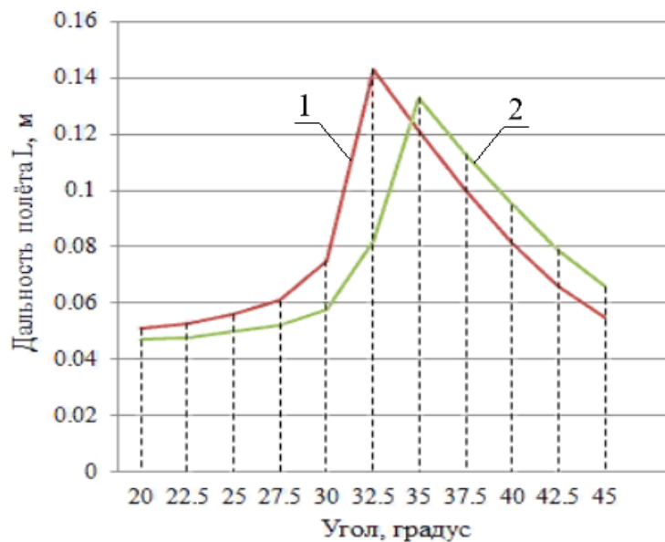
Рис. 3 – График зависимости дальности полёта частицы от углов наклона плоскостей распределителя при высоте падения h = 0,55 м:
