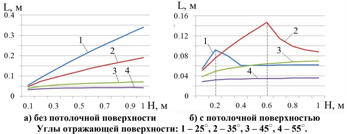
Рис. 2 – Графики зависимости дальности полёта частицы от высоты падения
